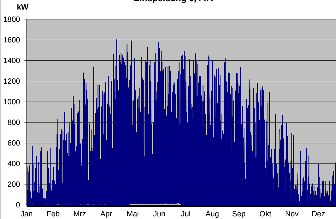
Einspeisung 0,4 kV
