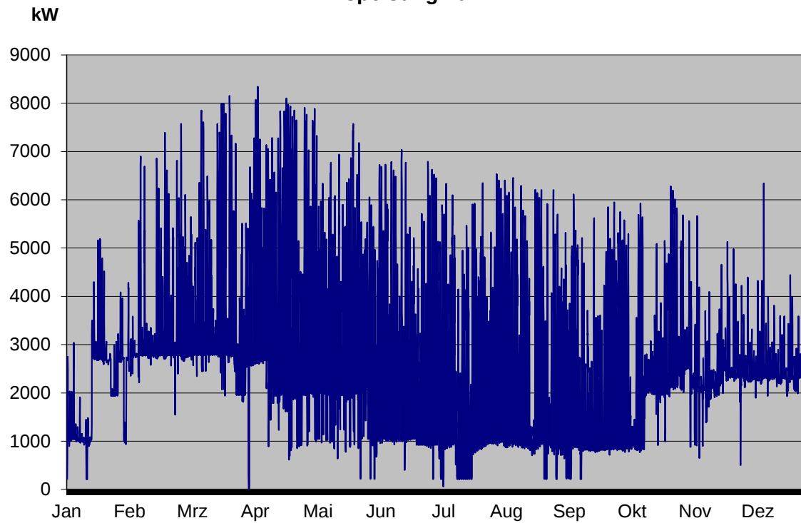
Einspeisung 20 kV
